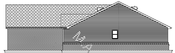
Right Elevation
